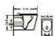
WH-028 مركب على الحائط Wall-hung toilet Size: 510x345x340mm الارتفاع: 340مم التركيب على الحائط: 180مم
