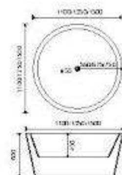
BT-054B جوشي استحمام قائم بذاته الحجم: 1100x1100x600 عمق: 600x1350x1350 بئر: 600x1500x1500
