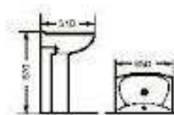
4025 حوض القاعدة الحجم: 650x510x820 مع مثبت على الحائط تثبيت على الحائط يظهر
