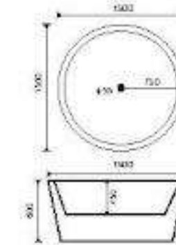
BT-058 جوشي استحمام قائم بذاته، الحجم: 1500x1500x600 عمق: 600x1350x1350
