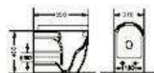
WH-003D مركب على الحائط Floor mounted toilet Size: 550x370x400mm الارتفاع: 400مم التركيب على الحائط: 180مم
